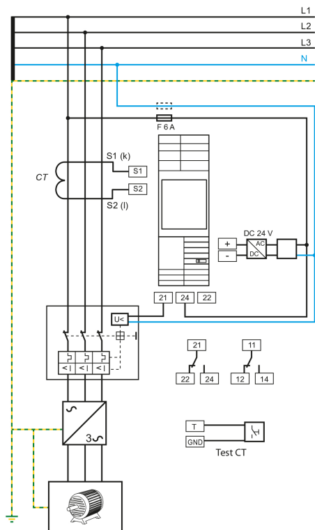
Anschlussbild Unterspannungsauslöser
